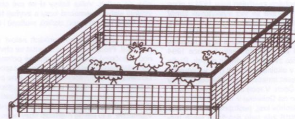
Obr. 3. pevný drátěný ohradník (výška min. 120 cm, lépe 140 cm), páska 20–30 cm nad ohradníkem opticky brání přeskocení ohrady, elektrický drát (min. 2 500 V) okolo ohrady cca 20 cm nad zemí brání podhrabání (proti podhrabání se dá také zapustit pevný drátěný ohradník min. 50 cm pod zem, nebo použít drátěné pletivo navazující na ohradník v úrovni země o šířce min. 100 cm)
